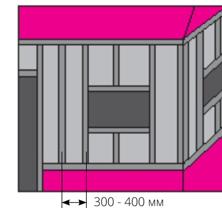
рис. 2 Вертикальная обрешетка
